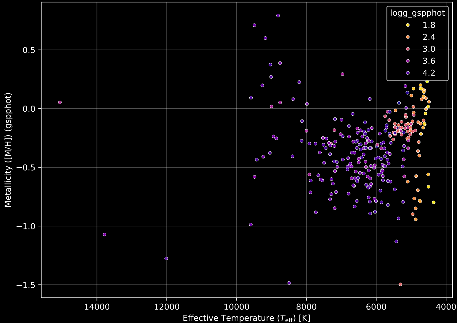
GALAH DR4 Field: [8960] Stellar Population Parameters (n= 277)
