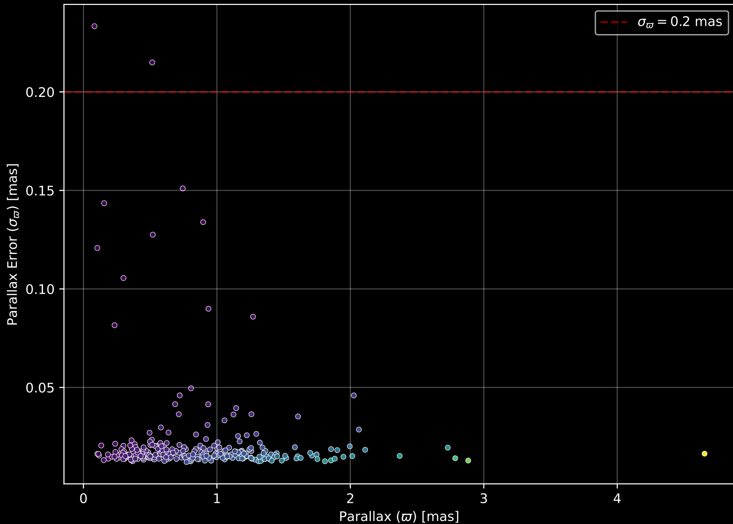
GALAH DR4 Field: [8960] Parallax Quality (n= 277)
