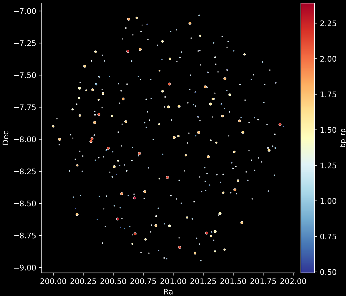
GALAH DR4 Field: [8960] Stars: 277
