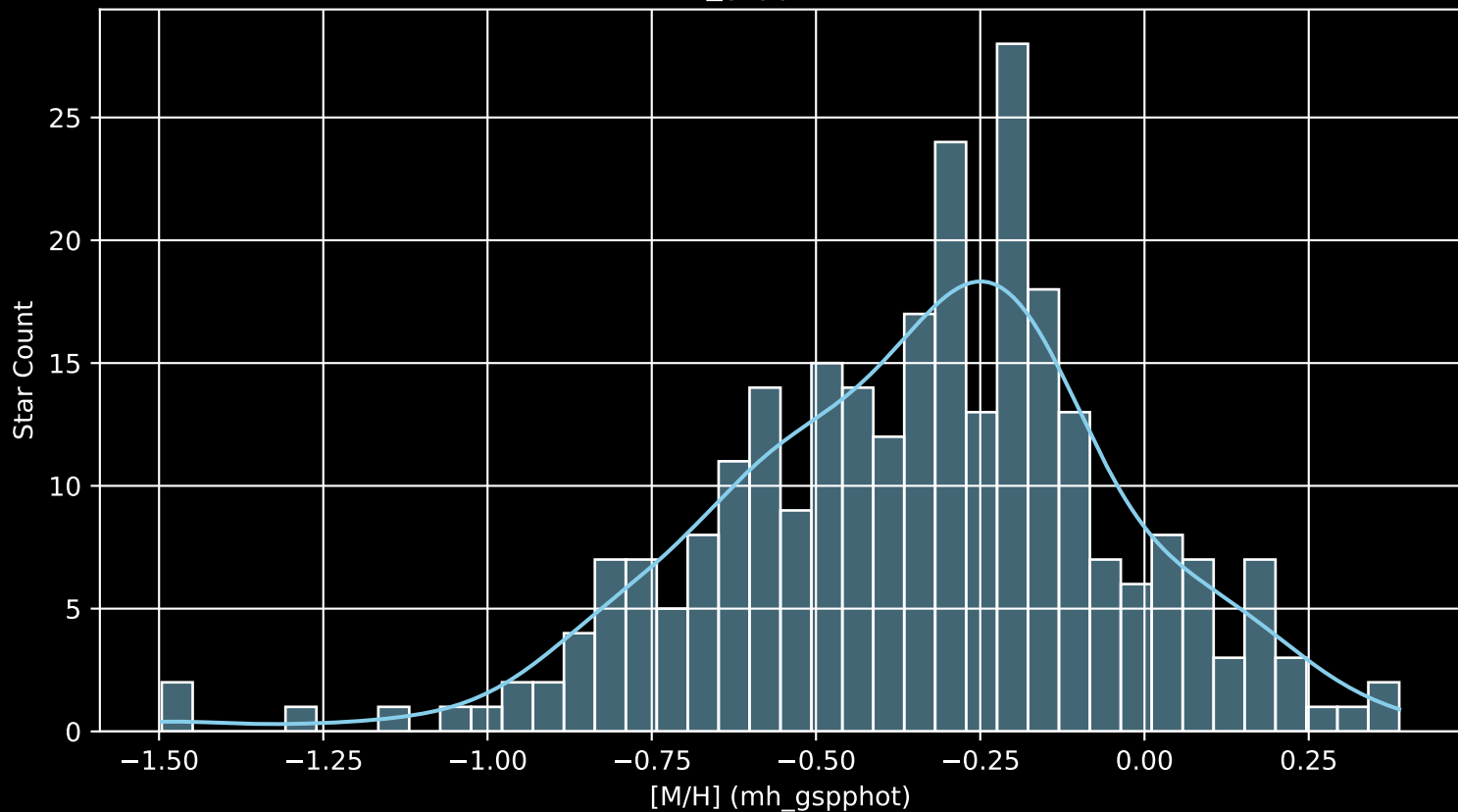
GALAH DR4 Field: [8960] [M/H] (mh_gspphot) (n= 274)
