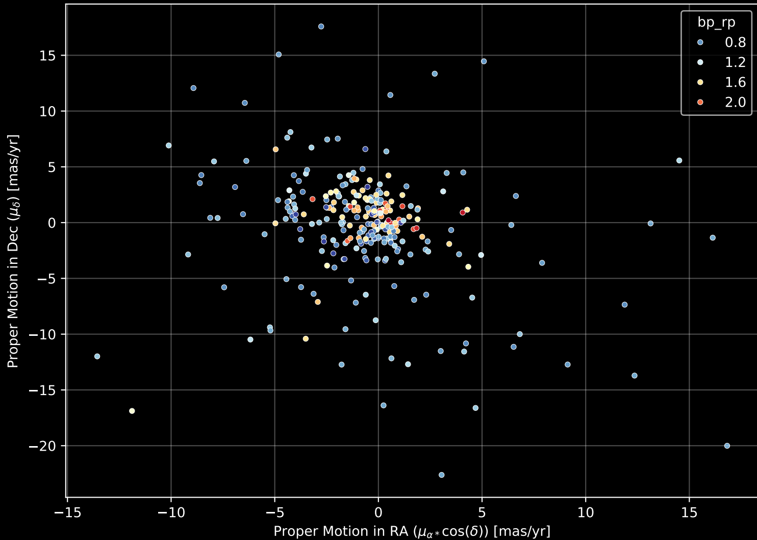
GALAH DR4 Field: [8960] Proper Motion Diagram (n= 277)
